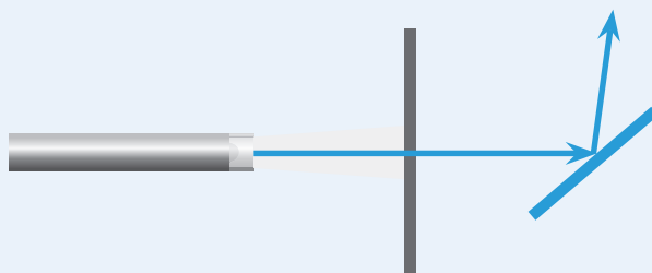
光在镜面上的反射示意图
