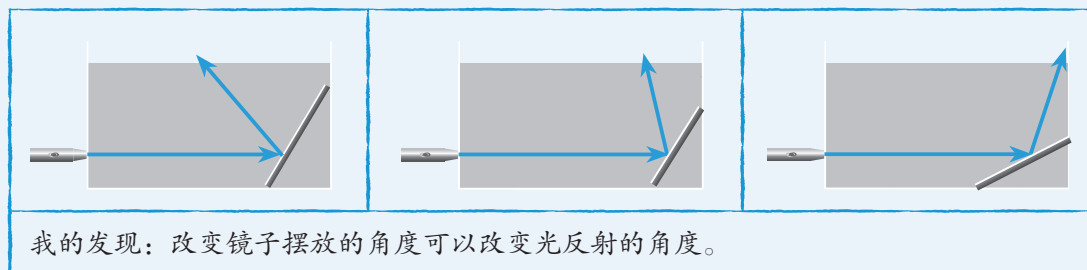
光在水槽里的镜面反射示意图
